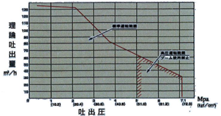
・NCP13FB-364理論性能グラフ
