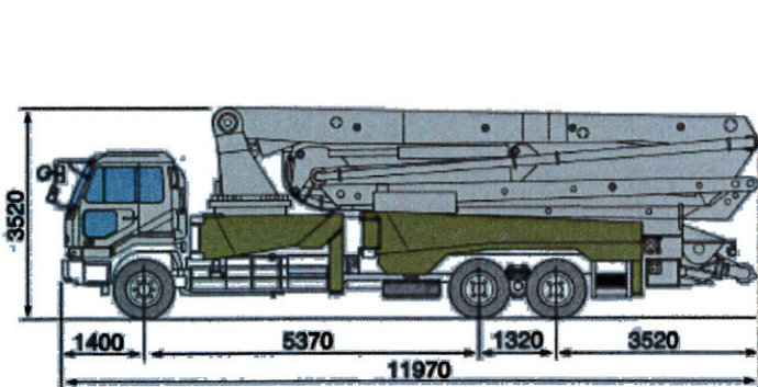
・NCP13FB-364外形図
